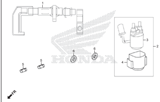
SET START MAG
