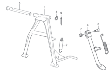
STAND
