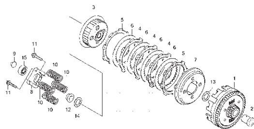
CLUTCH
