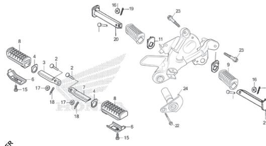
STEP
