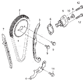
CAM CHAIN/TENSIONER
